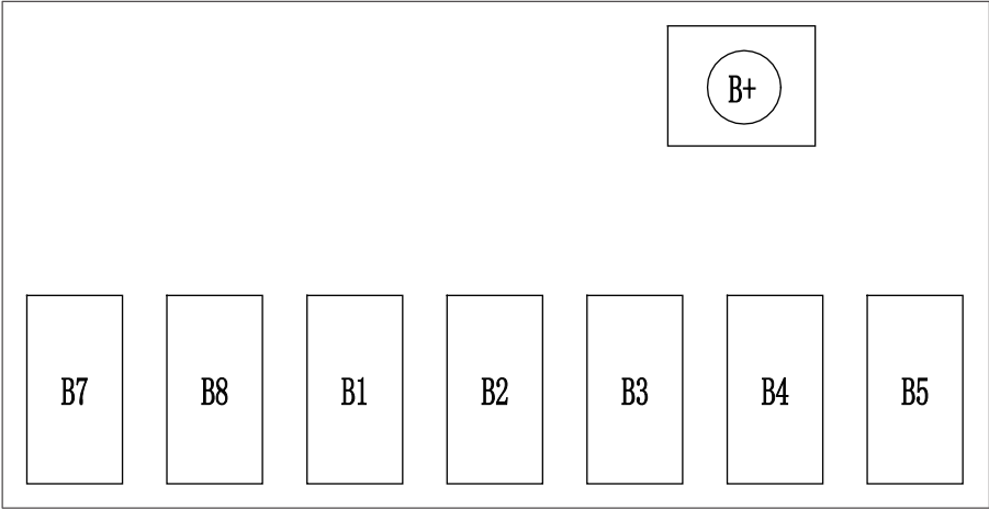
机舱蓄电池正极保险盒（装配激光雷达的车辆）
