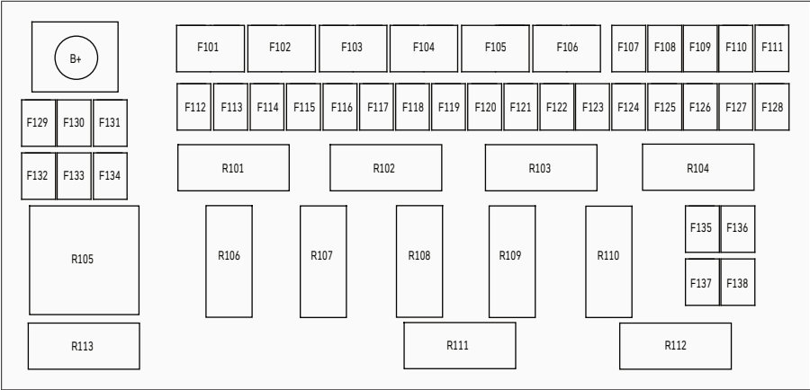
仪表保险盒
