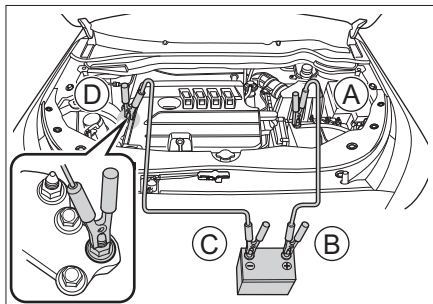
装配 GW4G15M 发动机的车辆
