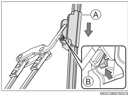
① 雨刮片 ② 弹性锁片
